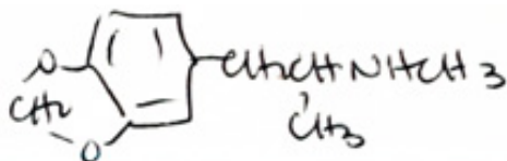
N-Me MDA. MDMA.
